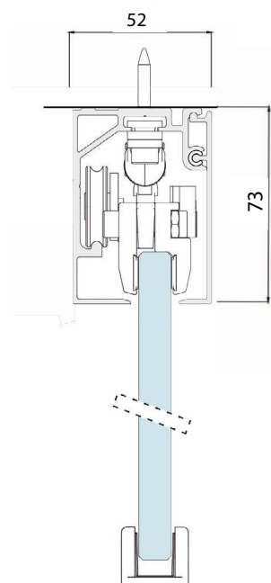
Fixation au plafond
