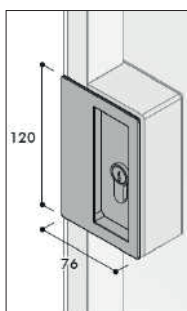
GEOD avec serrure à clé
