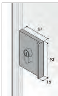
Serrure à clé
